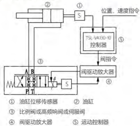
位置、速度控制原理图
