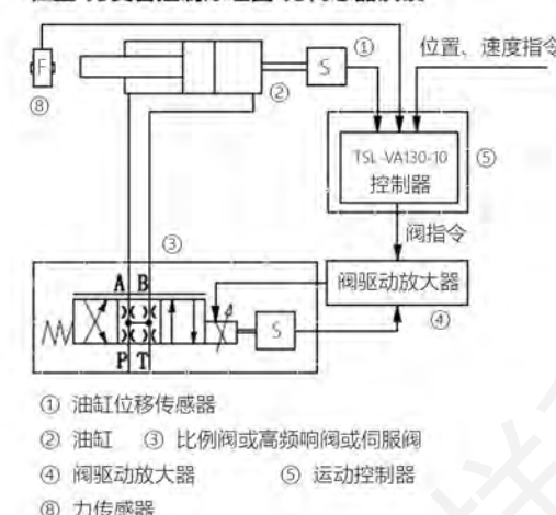
位置-力复合控制原理图-力传感器反馈
