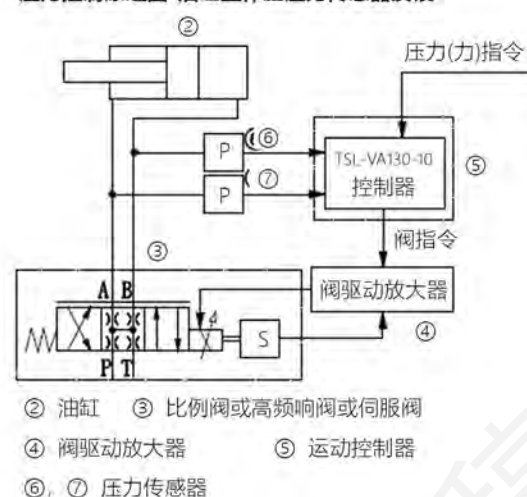
压力控制原理图-油缸工作腔压力传感器反馈
