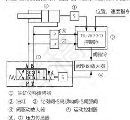
位置-压力复合控制原理图-油缸工作腔压力传感器反馈
