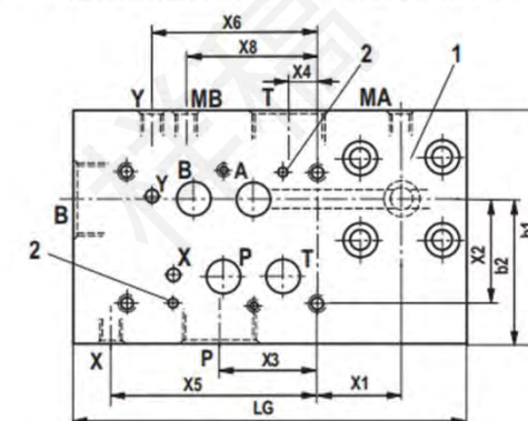
规格 16 油口安装面符合 ISO 24340 形式 A 和 ISO 4401
